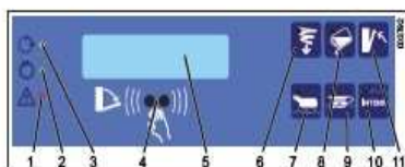
3. ábra: Vezérlőpanel
